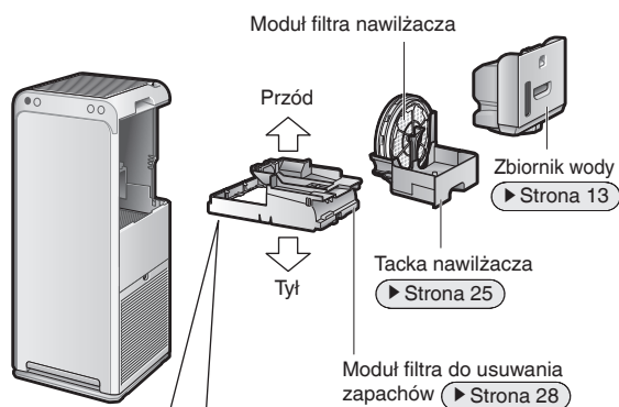
Tył modułu filtra do usuwania zapachów
