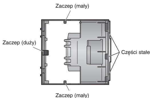
Tył modułu filtra do usuwania zapachów
